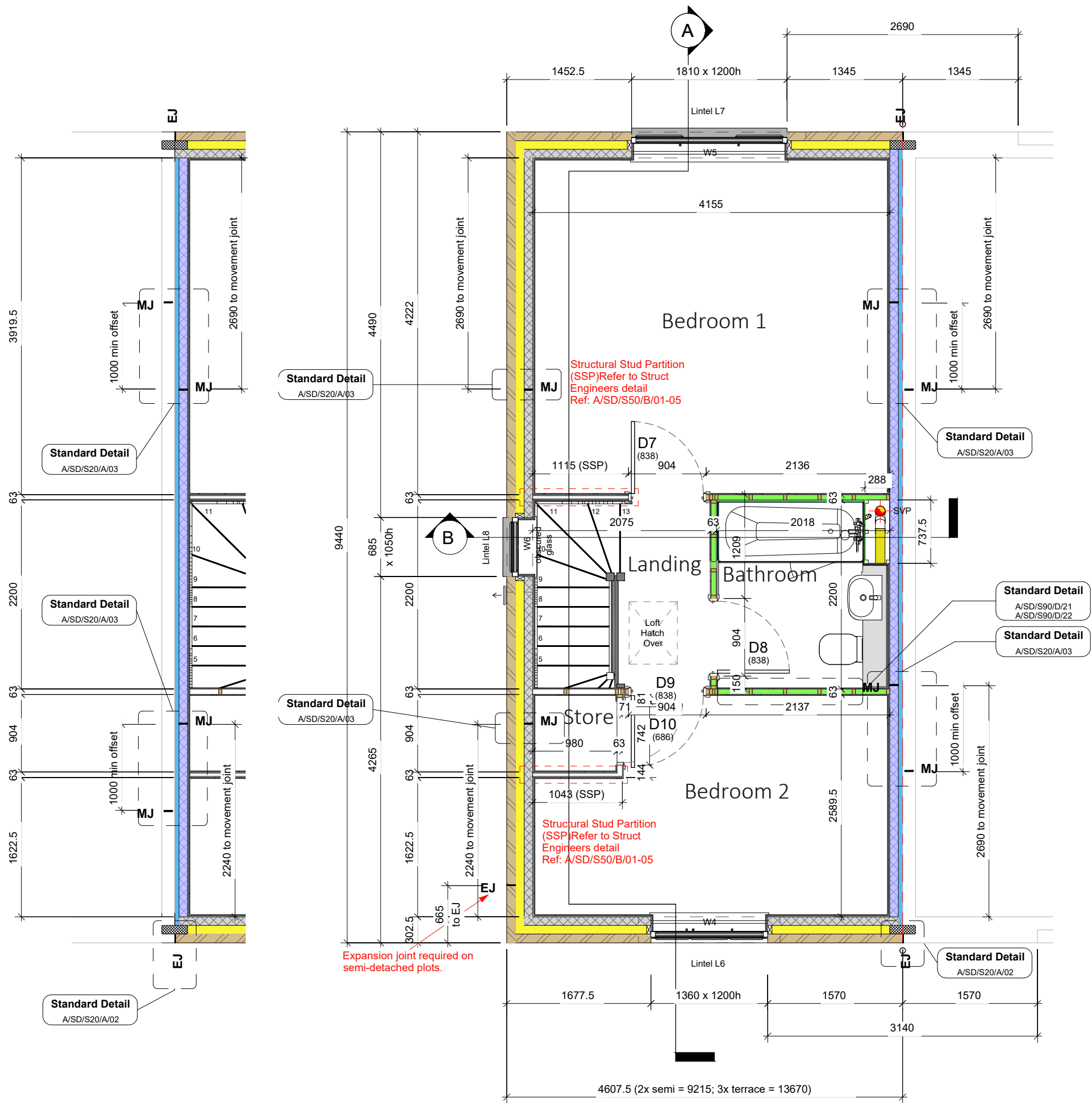
2 First Floor - Mid Tce 1 : 50
